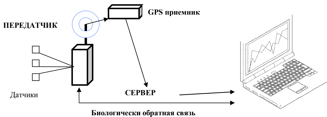
Рисунок 5 - Общая схема телеметрической системы
