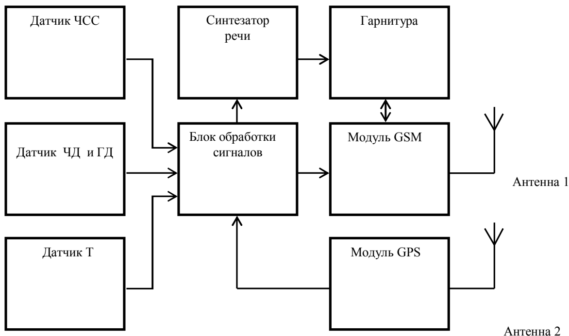
Рисунок 1 - Блок-схема телеметрической системы
