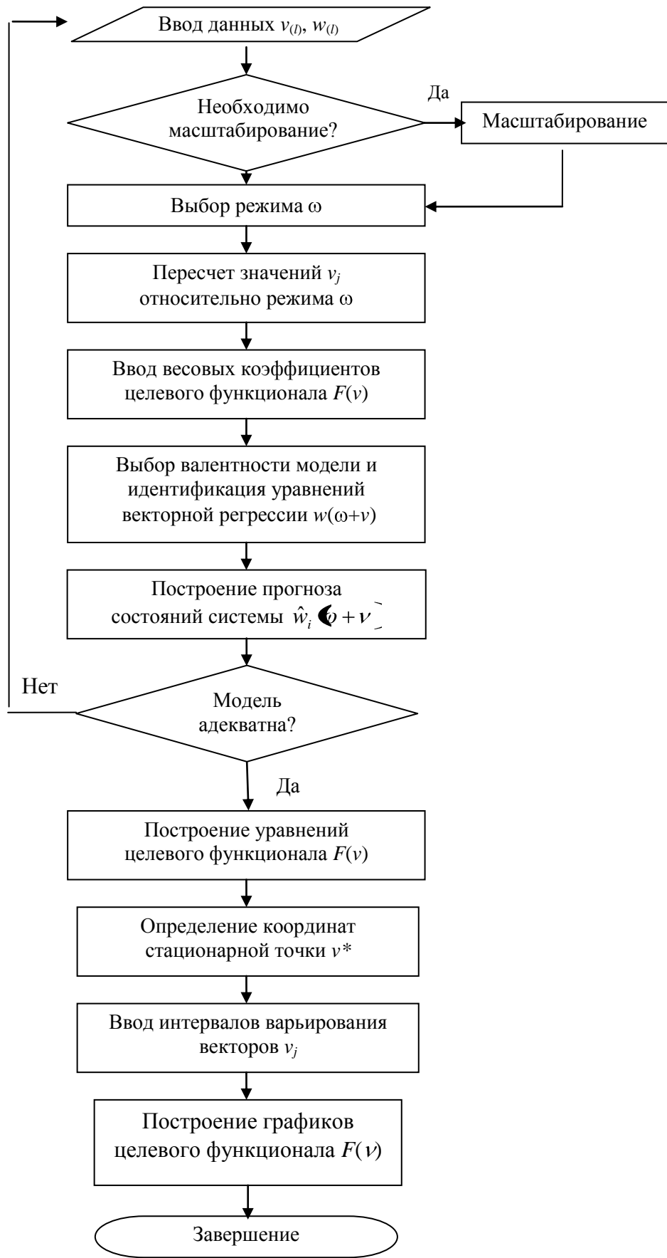
Рис.3.2. Алгоритм программного комплекса «ОРИЭП».
