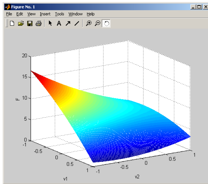
Рис. 3.19. Фрагмент целевого функционала F(v_1, v_2) в контуре квадрата Q
