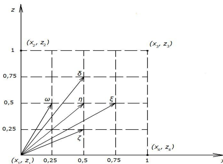
Рис. 3.10. Точки пеленгации (x_i, z_i) источника поля, обладающего координатами, определяемыми векторами \delta, \xi, \zeta, \eta, \omega
