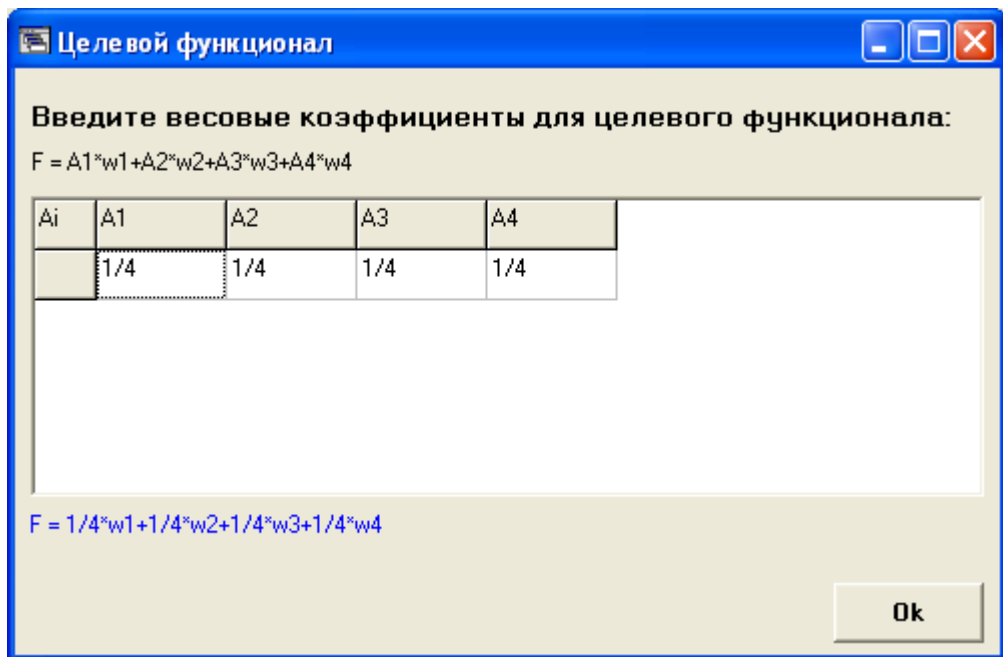
Рис. 3.8. Окно редактирования весовых коэффициентов
