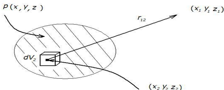
Рис. 3.1. Сплошное «пятно» распределения
