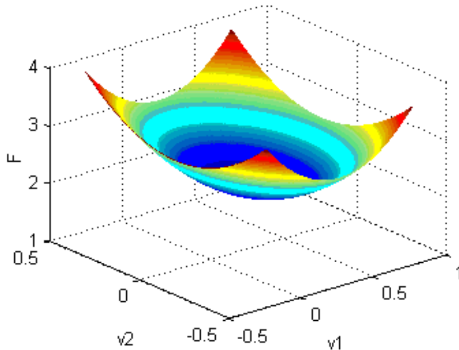
Рис. 3.11. Фрагмент целевого функционала F(v_1, v_2) в контуре квадрата Q
