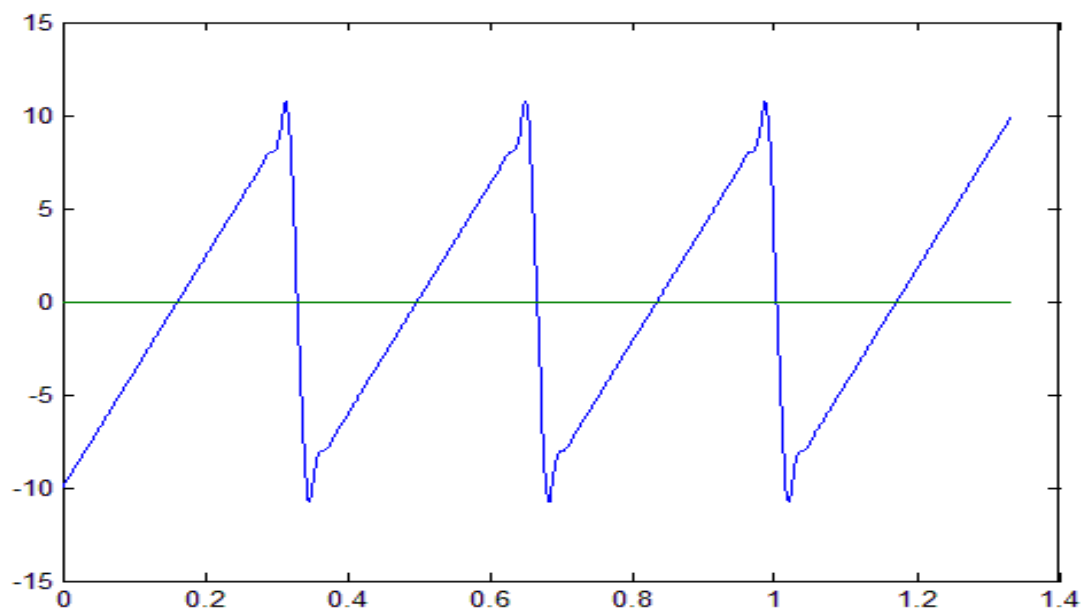
Рис. 3.23. График функции dF^\#(y)/dy .
