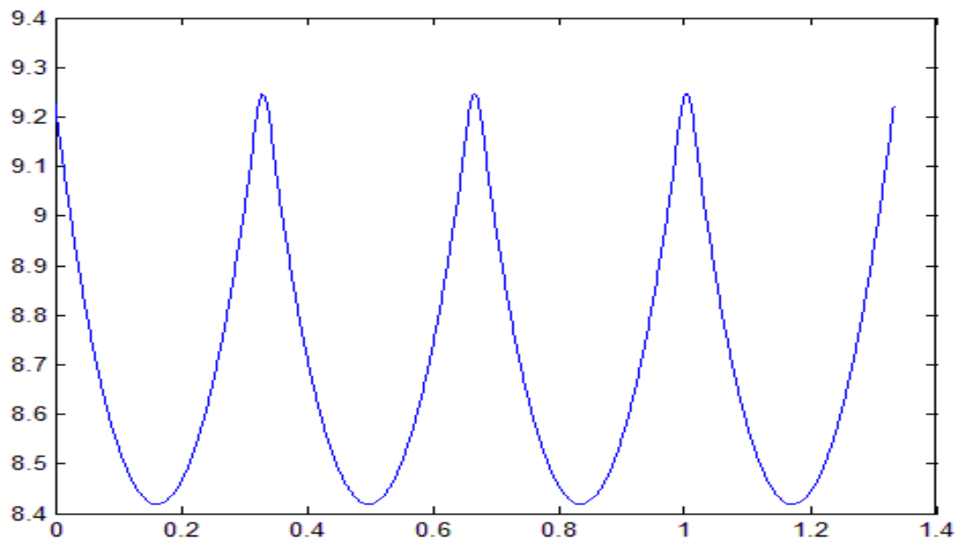
Рис. 3.22. График функции F^\#(y) .
