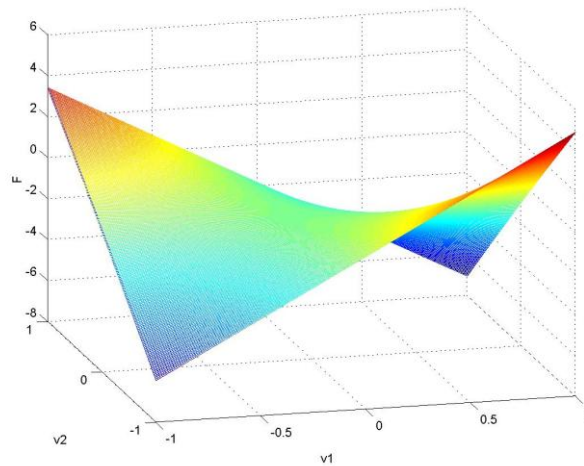
Рис. 3.15. Фрагмент целевого функционала F(v_1, v_2) в контуре квадрата Q
