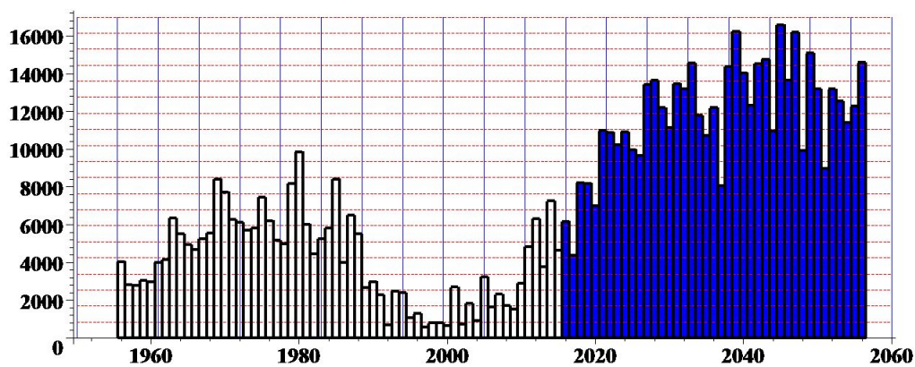
Рисунок 3.4 — Данные ввода генерирующих мощностей с 1956 по 2015 г. и стратегия вводов с 2016 по 2056 г. с ежегодным ростом располагаемой мощности на 2%, МВт
