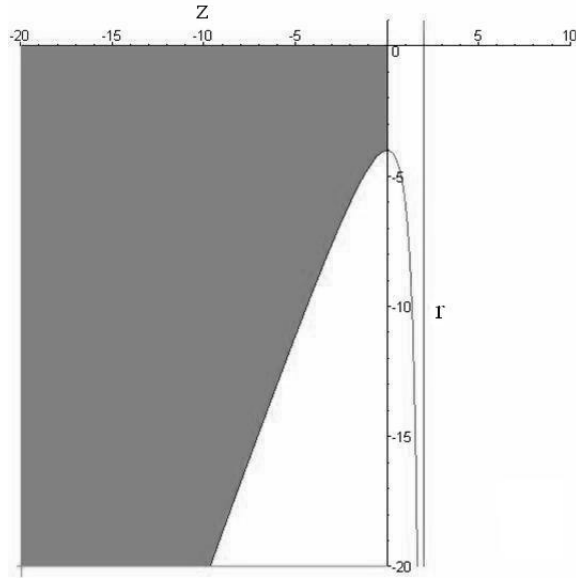
Рисунок 2.1 — Область устойчивости метода (2.19) для модельного примера (2.5) (заштрихована)
