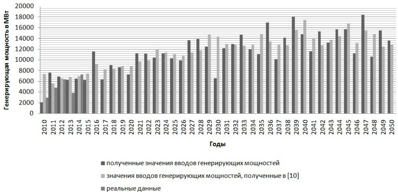
Рисунок 3.3 — Сравнение прогнозов ввода генерирующих мощностей с 2010 по 2050 г., темп роста располагаемой мощности — 2 % ежегодно
