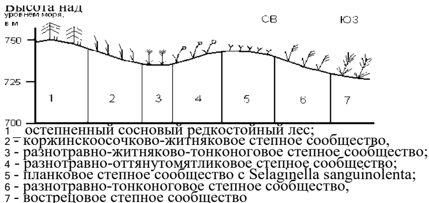
Рис. 16. Пример геоботанического профиля
