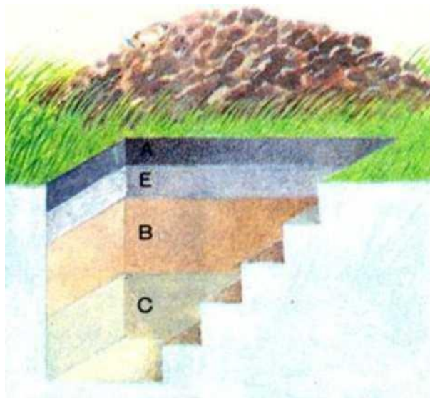
Рис. 4. Почвенный разрез
