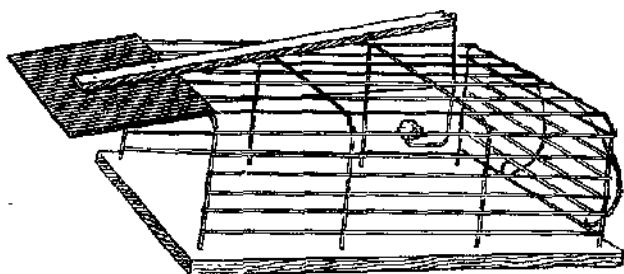
Рис.2. Мышеловка-живоловка (по Раллю)
